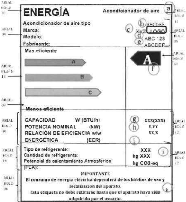
Figura N° 2 Características y contenido de la etiqueta.
